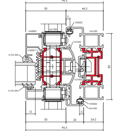
F82 LOCKING JAMB / C
